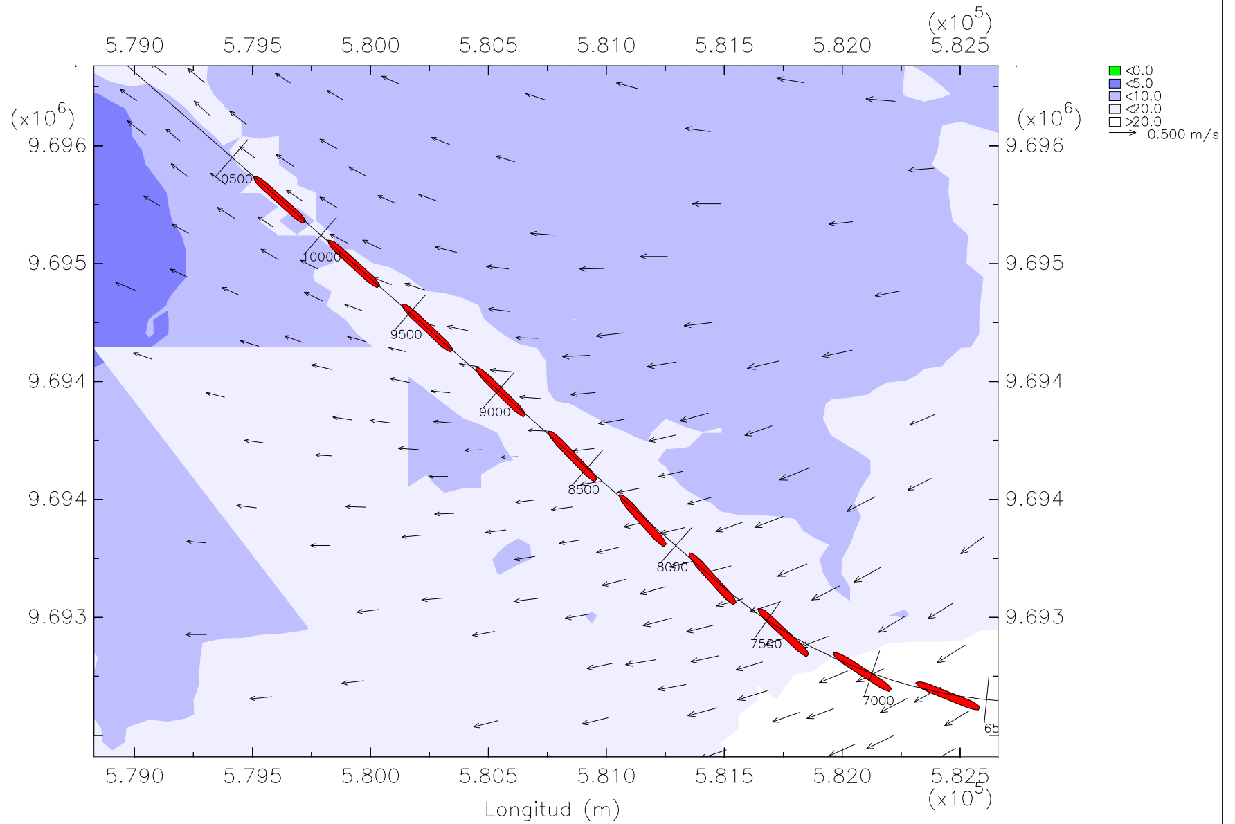
Z1T3 Trayectoria del barco portacontenedores panamax con corriente en reflujó
